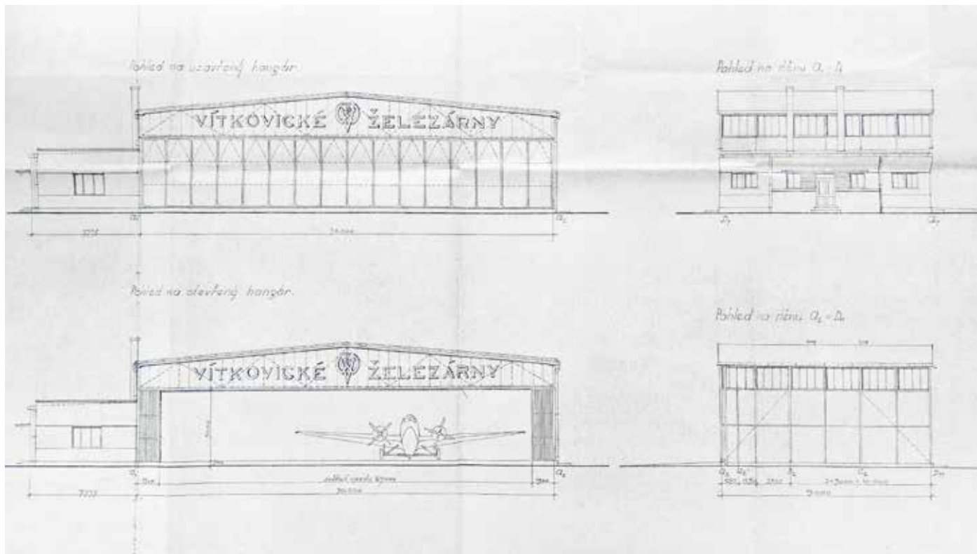
Stavební plány hangáru Vítkovických železáren z roku 1936
